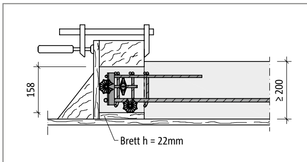
Schöck Tronsole® Typ Z: Herstellung einer Auflagerkonsole am Vollfertigteilpodest; Podestplattendicke h \geq 200 mm
