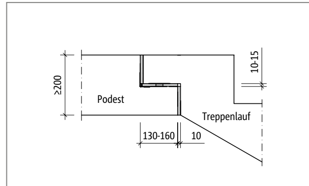
Schöck Tronsole® Typ F: Ausführungsvariante bündiger Treppenanschluss
