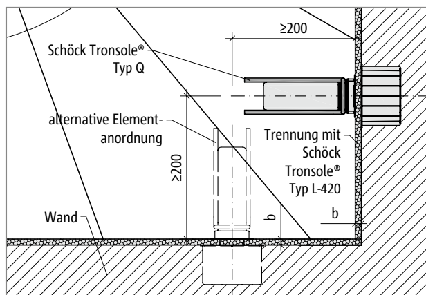
Schöck Tronsole® Typ Q: Elementanordnung, Detail A, Fugenbreite b = 15 mm bei Ortbeton, bei Fertigteiltreppenläufen ist die Notwendigkeit einer zusätzlichen Einbautoleranz durch den Planer zu prüfen
