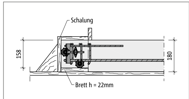
Schöck Tronsole® Typ Z: Herstellung einer Auflagerkonsole am Vollfertigteilpodest; Podestplattendicke h = 180 mm
