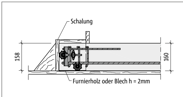
Schöck Tronsole® Typ Z: Herstellung einer Auflagerkonsole am Vollfertigteilpodest; Podestplattendicke h = 160 mm
