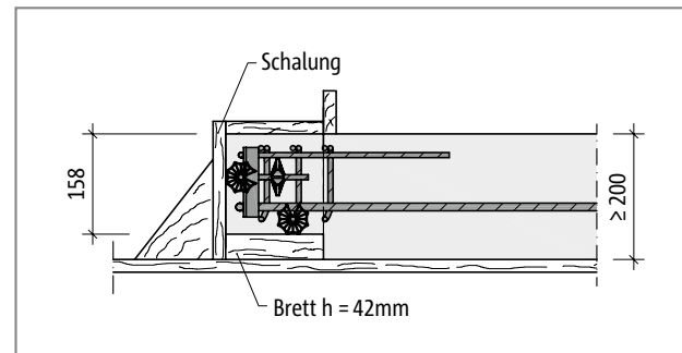
Schöck Tronsole® Typ Z: Herstellung einer Auflagerkonsole am Vollfertigteilpodest bei maximalem Höhenunterschied zwischen den Unterkanten des Podests und der Konsole; Podestplattendicke h \geq 200 mm
