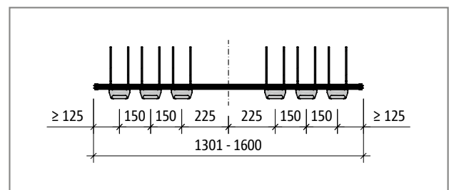
Schöck Tronsole® Typ T-V6-H...-L1301 bis L1600: Produktgrundriss
