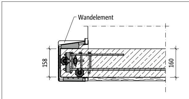
Schöck Tronsole® Typ Z: Wandelement als verlorene Schalung
