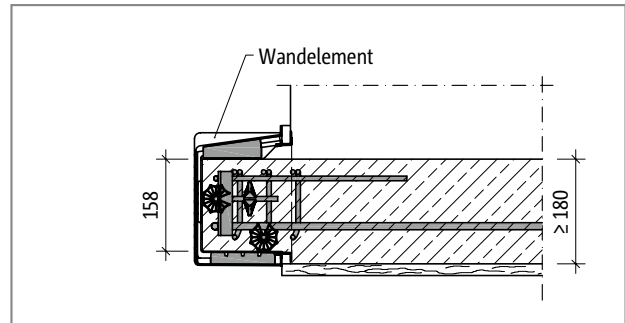
Schöck Tronsole® Typ Z: Wandelement als verlorene Schalung; Unterseite des Podests schließt bündig mit dem Anschlussrahmen des Wandelements ab.
