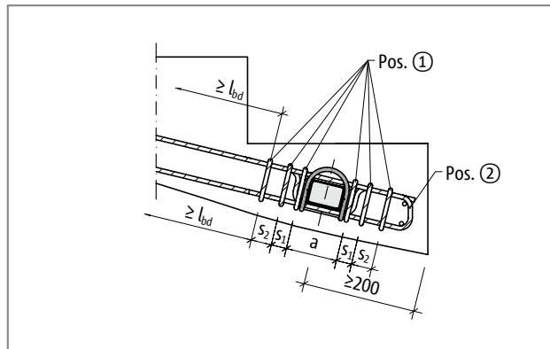
Schöck Tronsole® Typ Q: Ansicht „Fußpunkt“
