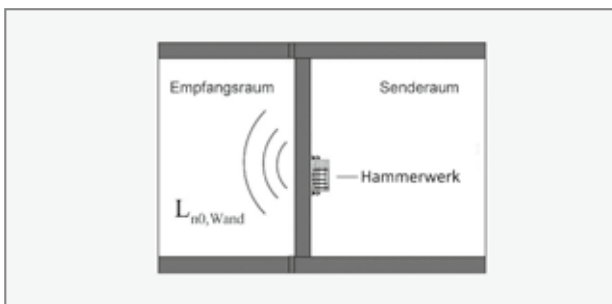
Bestimmung des Norm-Trittschallpegels L_{n0,Wand} im Schallprüfstand
